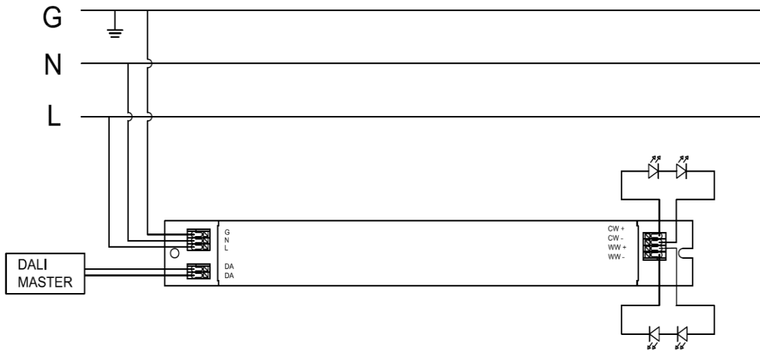
Fig.A:Dali Dimming
